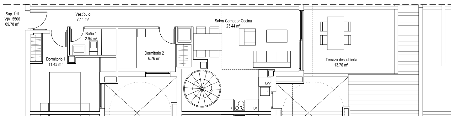
PLANTA INFERIOR
